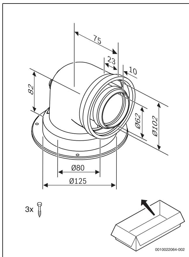
1 Ø 60/100: 7738112535
