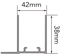
Perfil Profile
