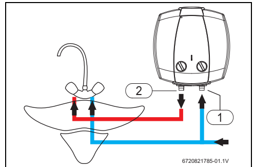
Fig. 8 Instalação por cima do lavatório
