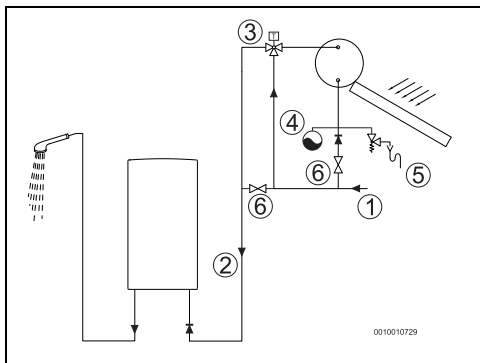
Fig. 19 Instalação solar
