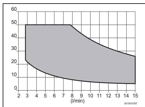
Fig. 31 Modelo 15 litros
