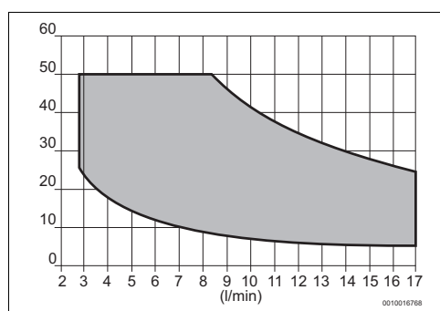
Fig. 32 Modelo 17 litros
