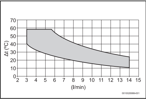
Fig. 31 Modelo 14 litros
