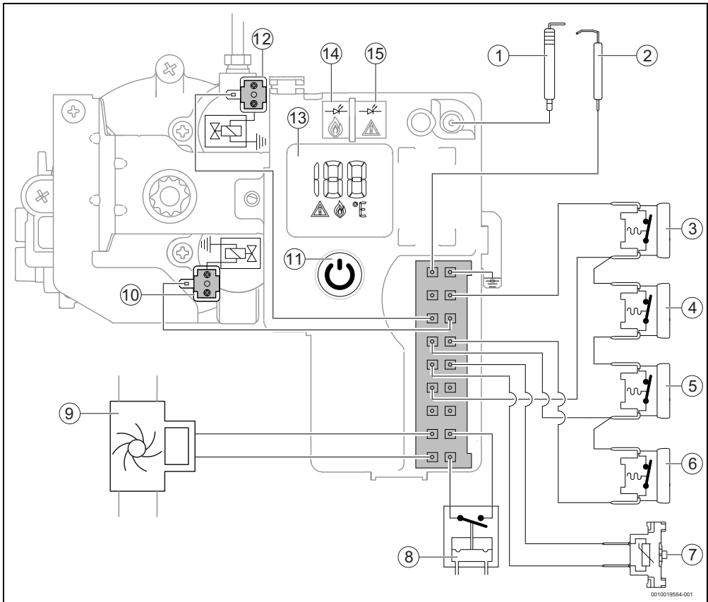
Fig. 29 Esquema elétrico
