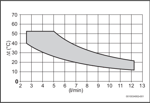
Fig. 30 Modelo 11 litros
