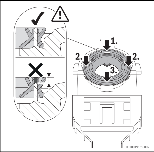
Fig. 52 Pressionar o vedante
