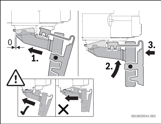
Fig. 53 Montar a recolha de condensados
