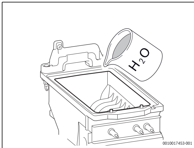
Fig. 48 Purgar o bloco térmico
