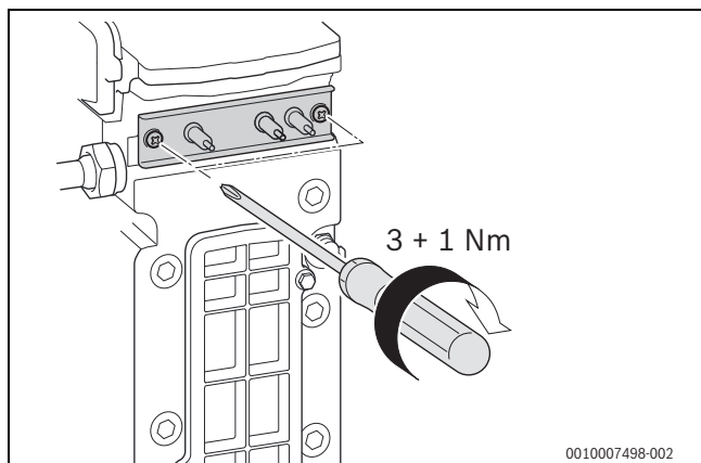
Fig. 38 Instalar o conjunto de létrodo
