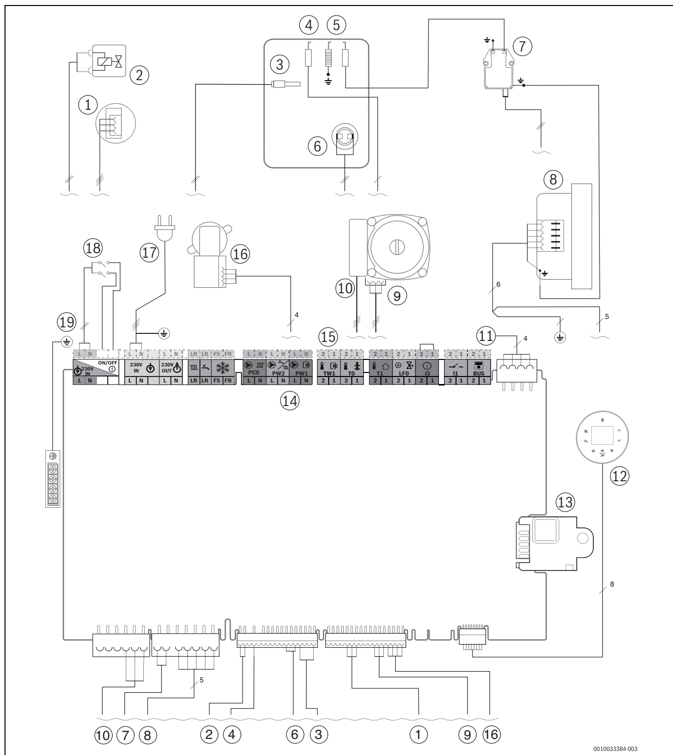
Fig. 62 Cablagem elétrica
