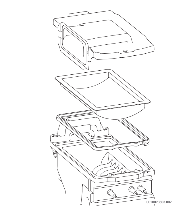
Fig. 41 Queimador
