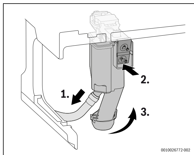
Fig. 50 Desmontar a recolha de condensados
