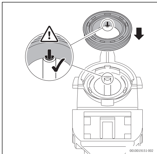
Fig. 51 Alinhar corretamente o novo vedante recolha de condensados
