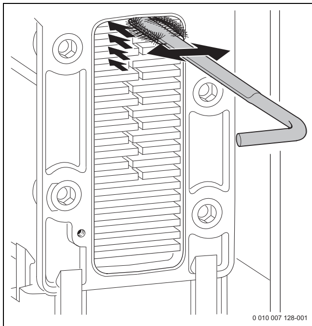
Fig. 47 Limpar o bloco térmico com a escova
