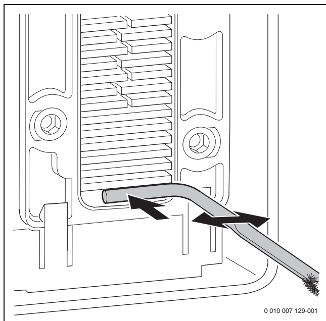
Fig. 49 Limpar a cuba de condensados
