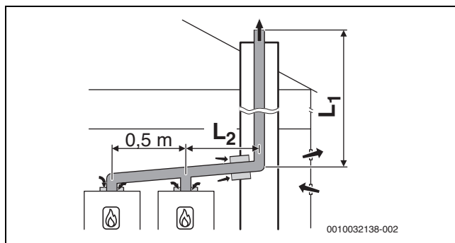
Fig. 13 Cascata com 2 aparelhos:
