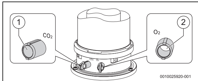
Fig. 29 Porto de medição de gases queimados e ponto de medição do ar de combustão
