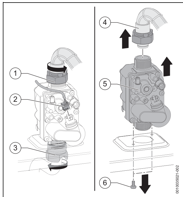
Fig. 48 Remoção da válvula de gás
