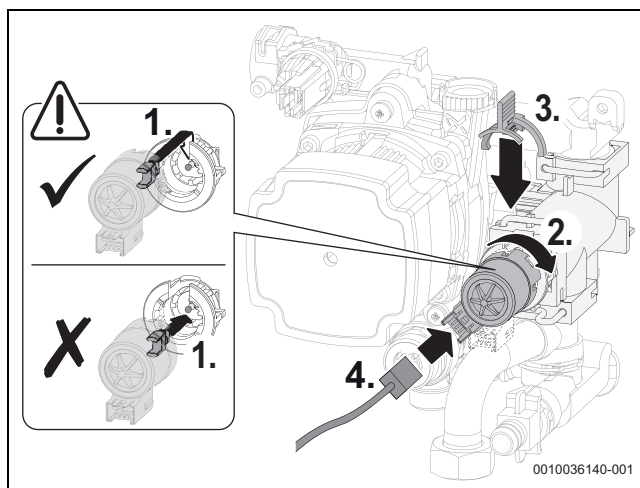
Fig. 50 Instalação do motor na válvula de 3 vias (variante sem parafusos)
