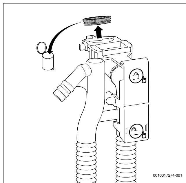
Fig. 43 Remoção da vedação no topo da recolha de condensados
