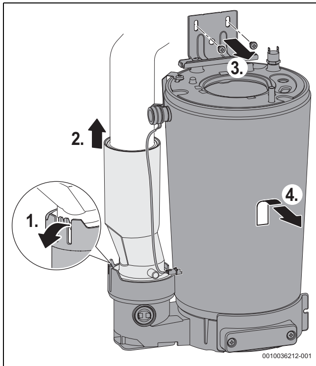
Fig. 54 Desmontar o conjunto do permutador de calor
