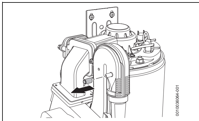
Fig. 47 Teste o bocal roscado no dispositivo de mistura
