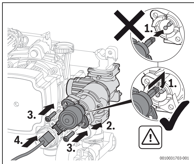
Fig. 52 Instalação do motor na válvula de 3 vias (variante com parafusos)
