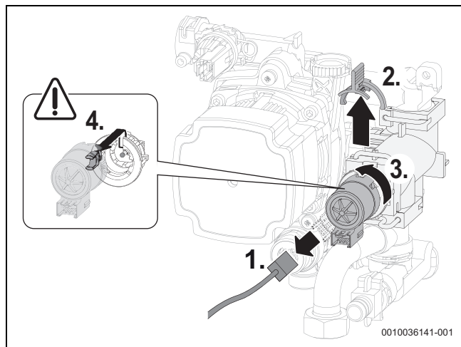
Fig. 49 Soltar o motor da válvula de 3 vias (variante sem parafusos)
