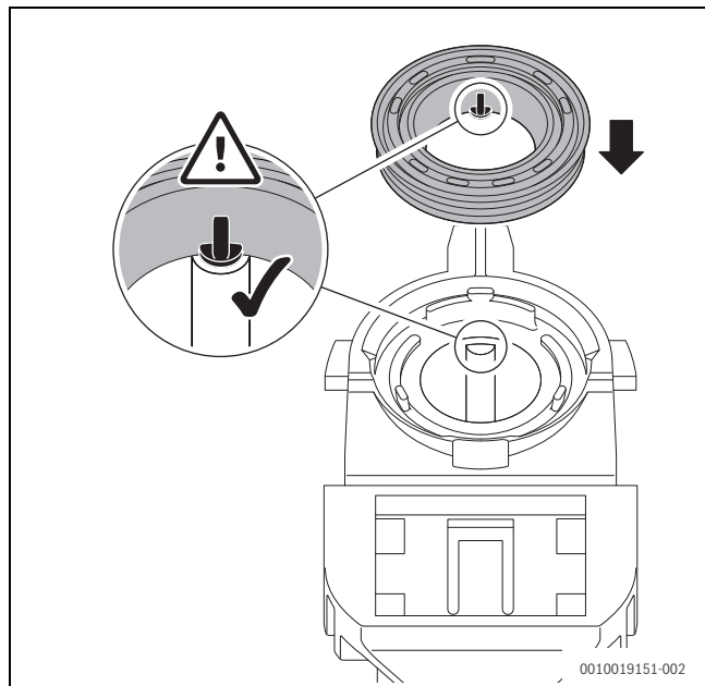
Fig. 44 Alinhamento da vedação com a recolha de condensados
