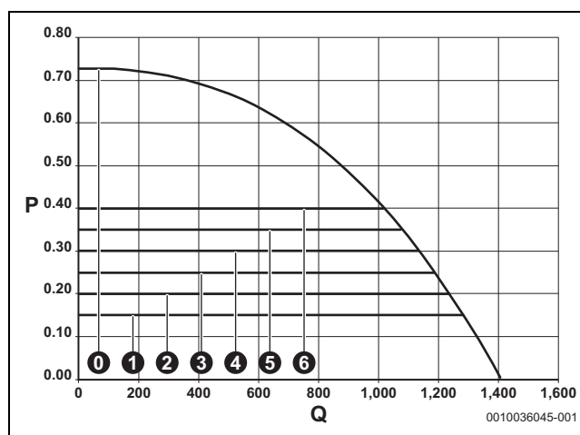
Fig. 57 Campos de funcionamento da bomba e curvas características da bomba
