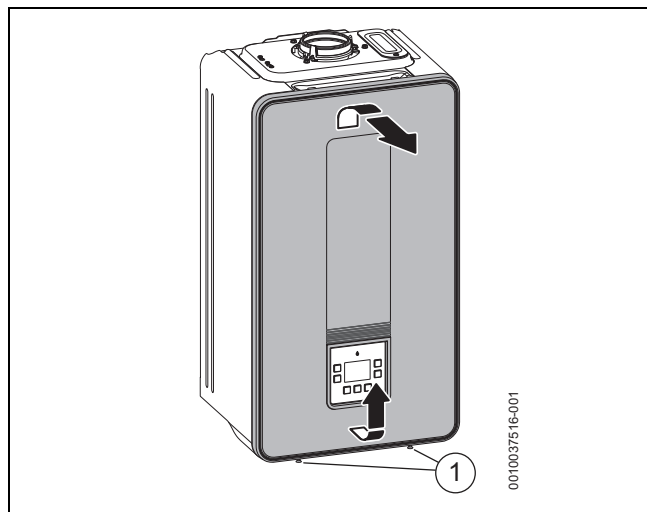
Fig. 27 Remoção do revestimento frontal
