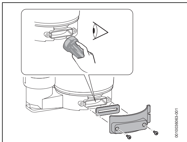
Fig. 40 Verificação do permutador de calor quanto a resíduos
