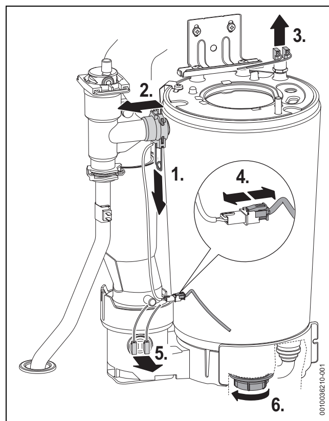
Fig. 53 Separação de componentes do conjunto do permutador de calor
