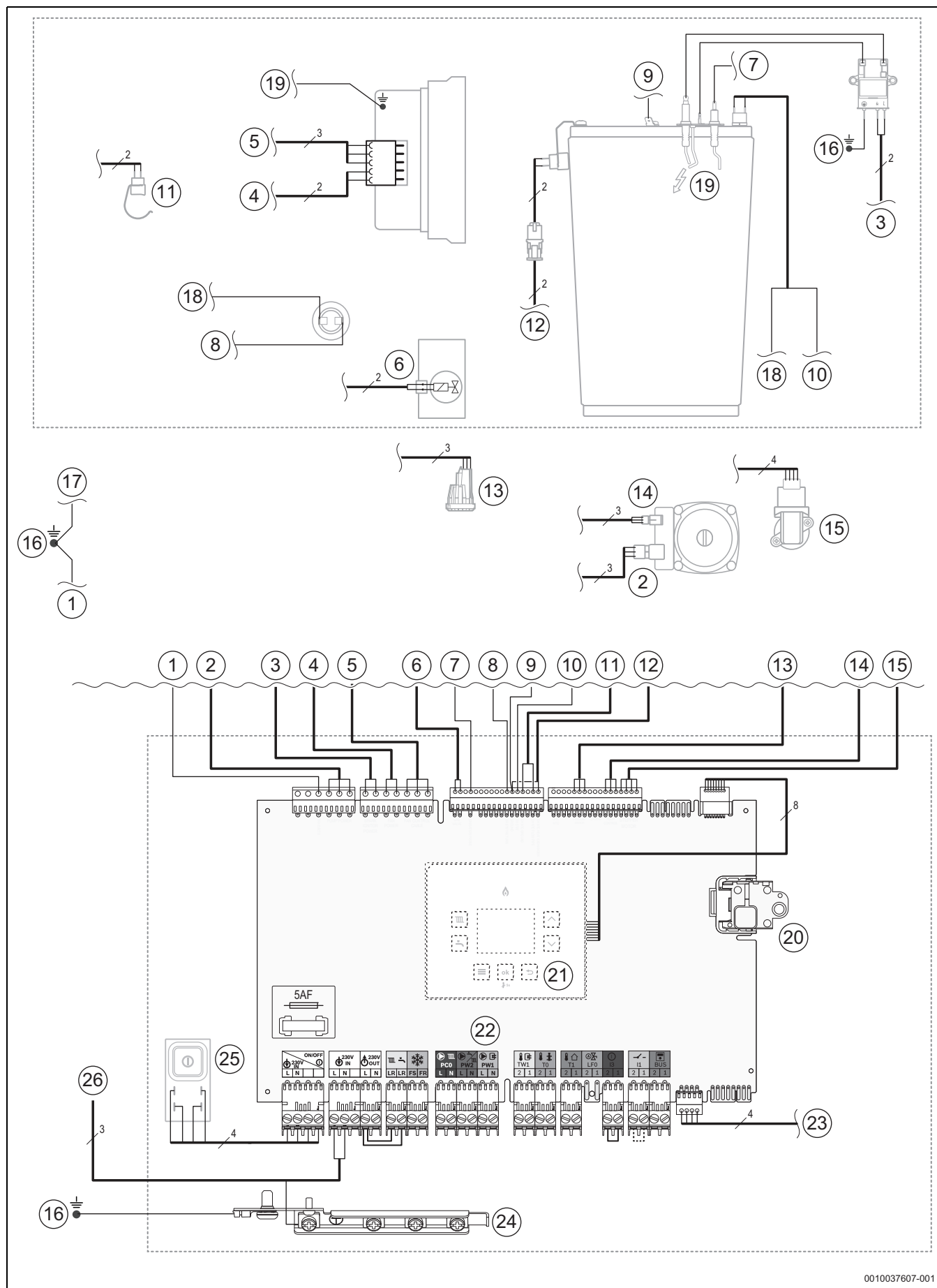
Fig. 58 Cablagem elétrica
