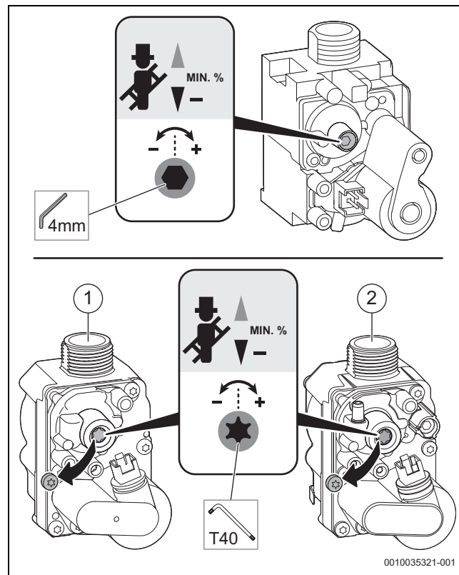
Fig. 30 Definição do teor de CO 2 ou O 2
