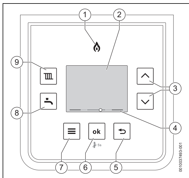
Fig. 26 Painel de comandos
