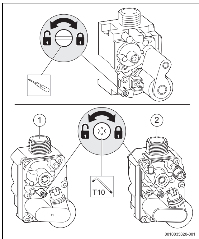
Fig. 28 Verificação da pressão de alimentação de gás
