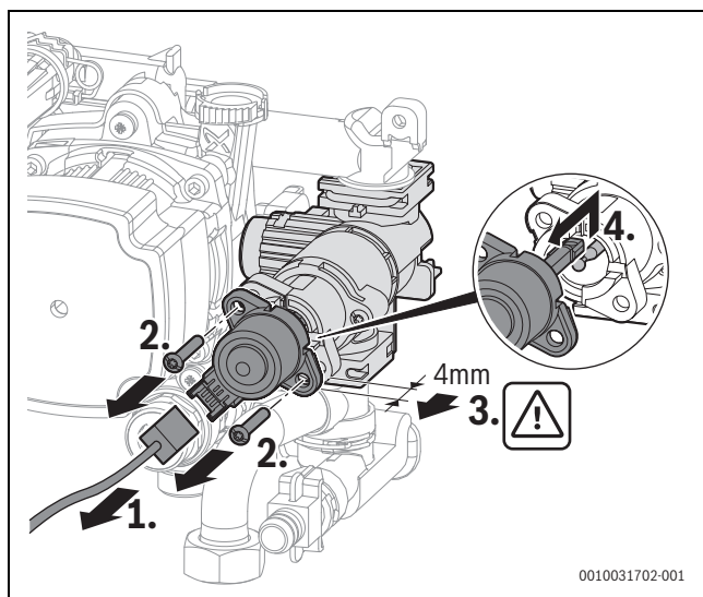
Fig. 51 Soltar o motor da válvula de 3 vias (variante com parafusos) Instalação do motor.
