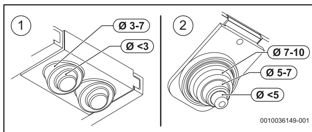
Fig. 21 Adaptar as buchas ao diâmetro do cabo
