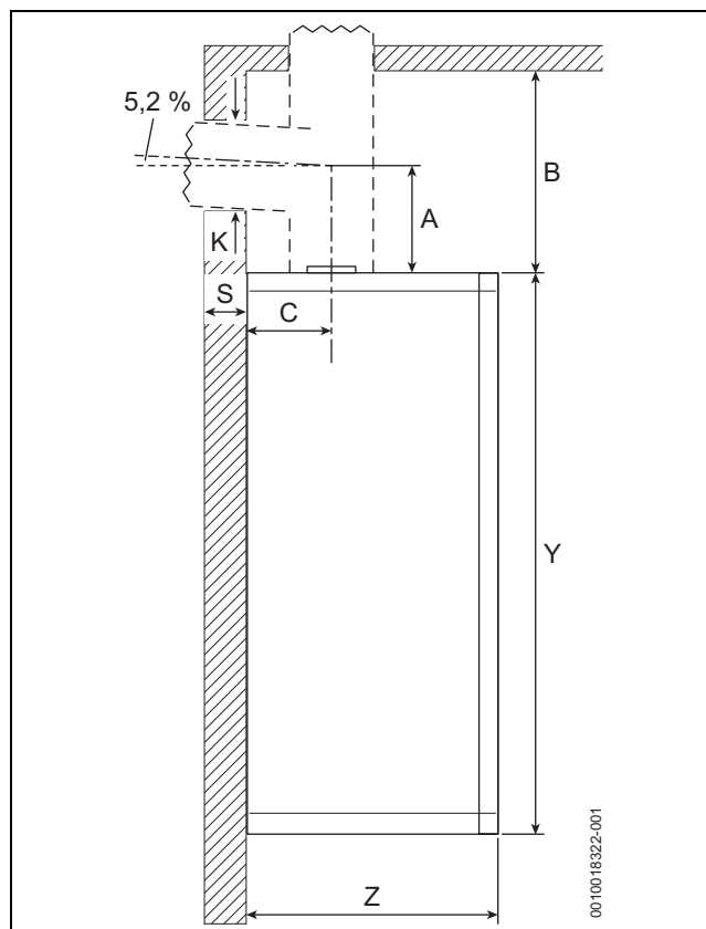
Fig. 2 Vista lateral
