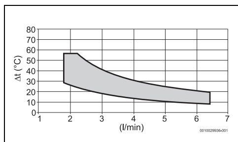
Fig. 28 Modelo 5 litros
