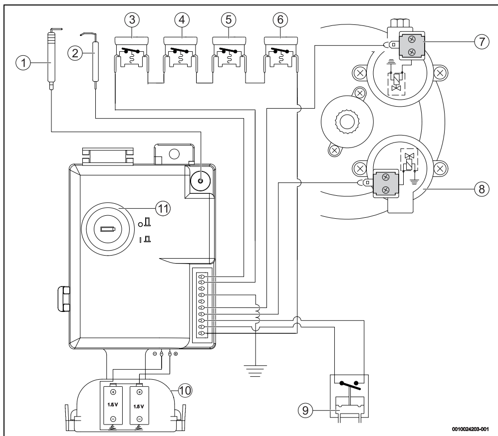
Fig. 27 Esquema elétrico
