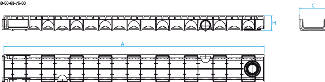
SAÍDA INFERIOR Ø40-50-63-75-80
