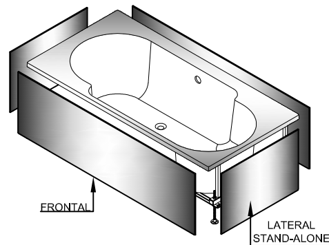
APLICAÇÃO STAND-ALONE (Painel frontal+painel lateral stand-alone)
