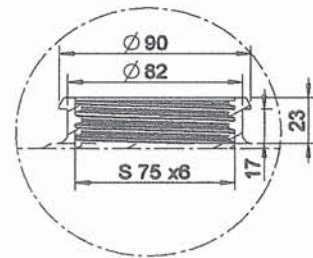
Detalle A sin tapón
