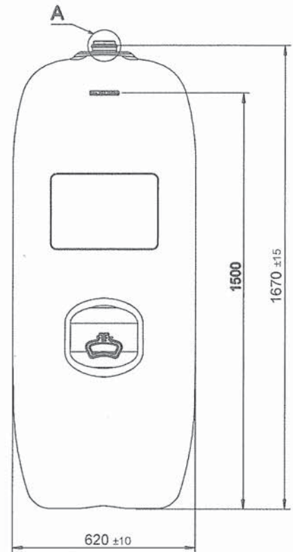
Detalle A sin tapón
