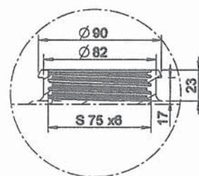
Detalle A sin tapón
