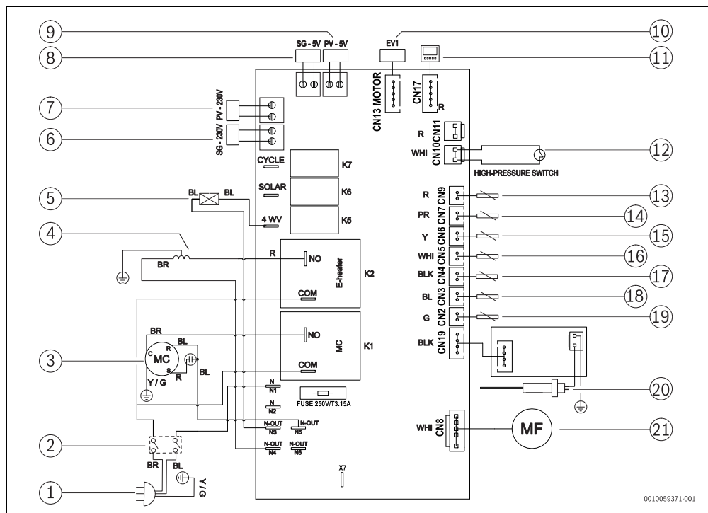
Fig. 33 Diagrama elétrico
