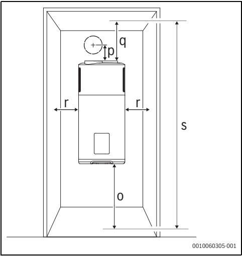
Fig. 9 Distâncias mínimas sem estrutura de suporte
