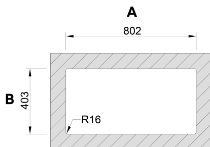
Instalação Inferior
