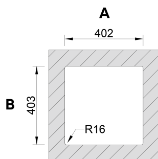
Instalação Inferior
