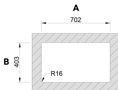
Instalação Inferior
