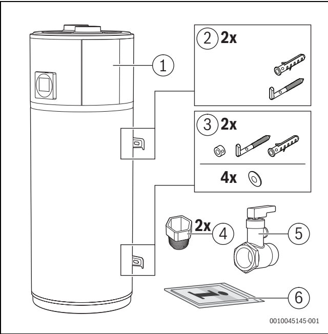
Fig. 1 Equipamento fornecido
