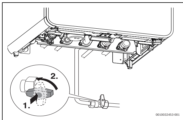
Fig. 5 Abrir a torneira do gás
