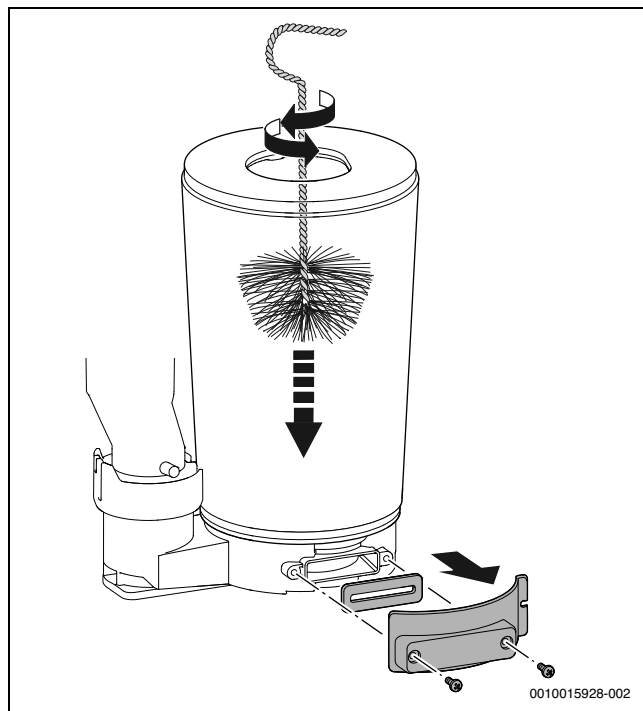
Fig. 47 Limpar o bloco térmico
