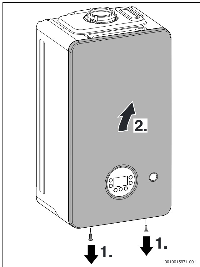
Fig. 22 Retirar o revestimento frontal
