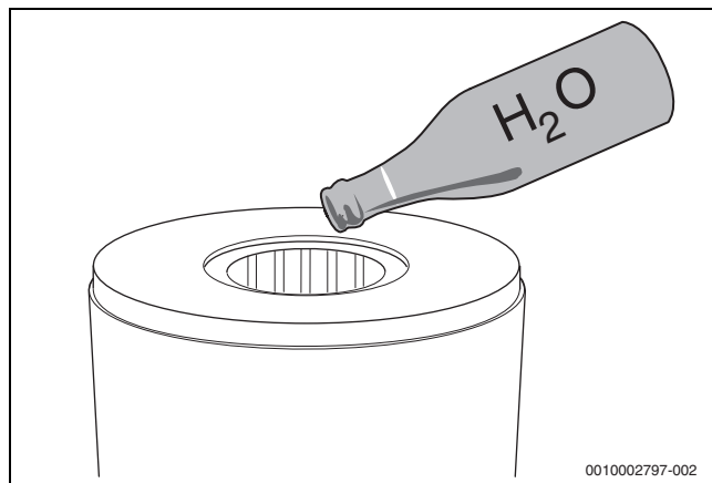
Fig. 49 Lavar o bloco térmico com água
