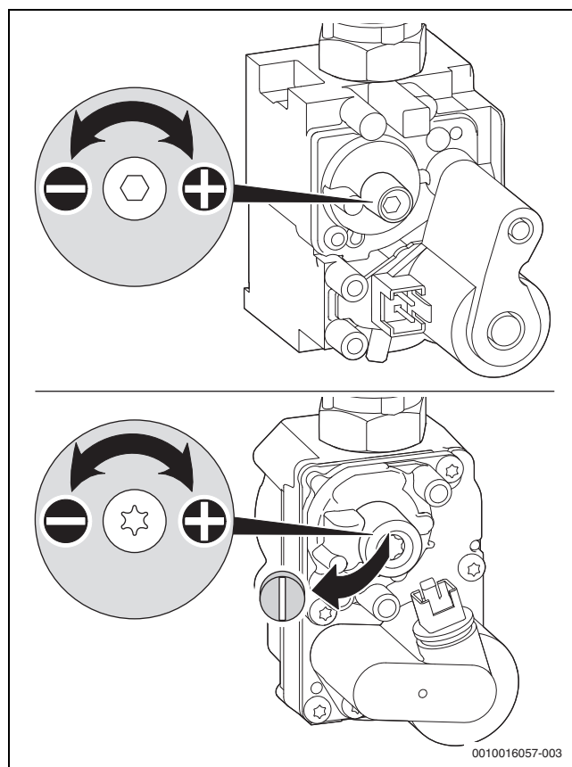
Fig. 36 Retirar o selo de chumbo do parafuso de ajuste
