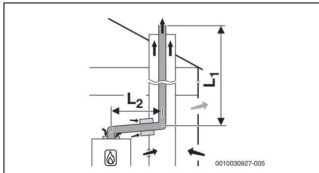
Fig. 14 Tubagem rígida de gases queimados no compartimento de acordo com B 53p com ar de admissão dependente do ar ambiente no aparelho e tubo de gases queimados simples no local de instalação; abertura de ventilação traseira no compartimento
