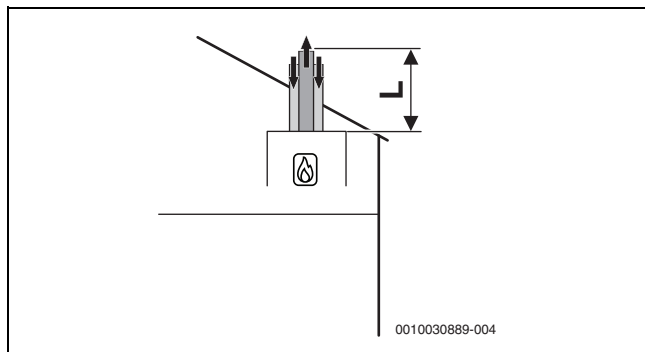
Fig. 9 Condução vertical e concêntrica dos gases queimados para o exterior de acordo com C 33x
