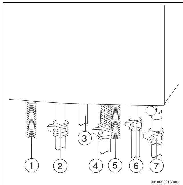
Fig. 25 Ligações do lado do gás e da água (acessórios)
