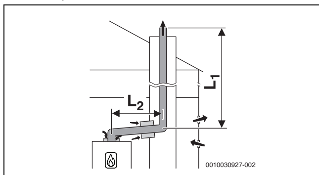
Fig. 16 Tubagem rígida de gases queimados na conduta de acordo com B 23p /B 53p com ar de admissão dependente do ar ambiente no aparelho e peça de ligação concêntrica entre o local de instalação e a conduta
