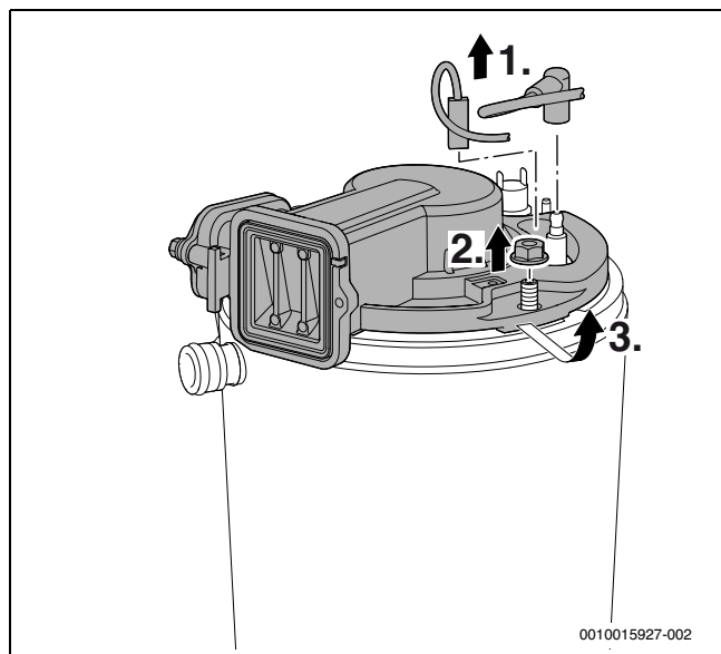
Fig. 42 Soltar a tampa do queimador
