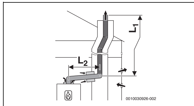
Fig. 17 Tubagem flexível de gases queimados na conduta de acordo com B 23p /B 53p com ar de admissão dependente do ar ambiente no aparelho e peça de ligação concêntrica entre o local de instalação e a conduta
