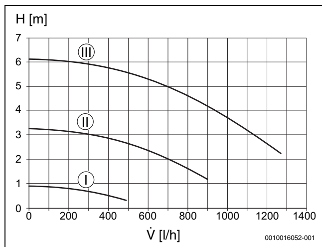
Fig. 32 Curva característica da bomba circuladora (rotações constantes)
