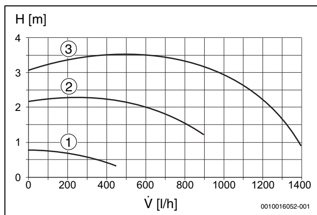
Fig. 34 Curva característica da bomba circuladora (pressão proporcional)
