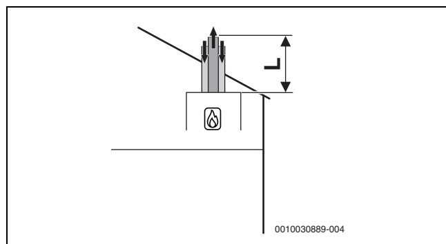
Fig. 7 Condução vertical e concêntrica dos gases queimados para o exterior de acordo com C_{33x}
