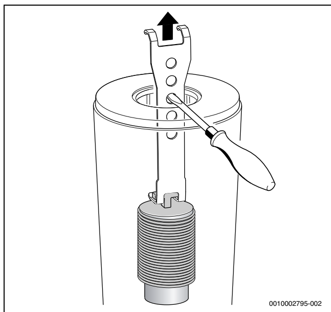
Fig. 46 Retirar o corpo de deslocamento inferior
