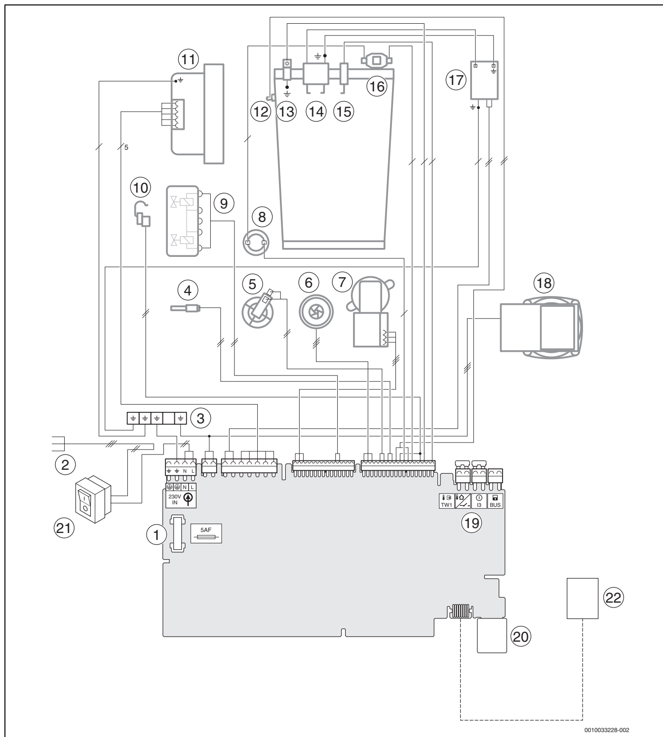
Fig. 71 Cablagem elétrica
