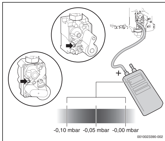
Fig. 35 Inspeção da pressão diferencial
