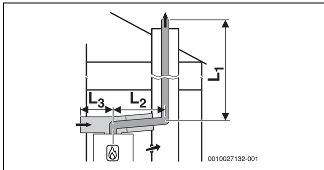
Fig. 12 Condução de gases queimados rígida de acordo com C 53x no compartimento e condução dos gases de escape para o exterior com tubos separados para ar de admissão e escoamento concêntrico de gases queimados no local de instalação
