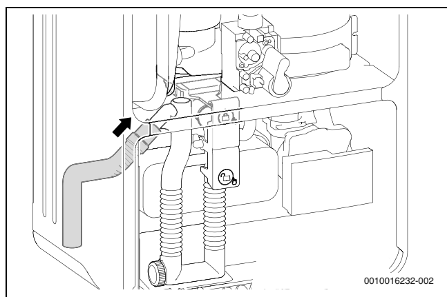
Fig. 24 Montar a mangueira na recolha de condensados
