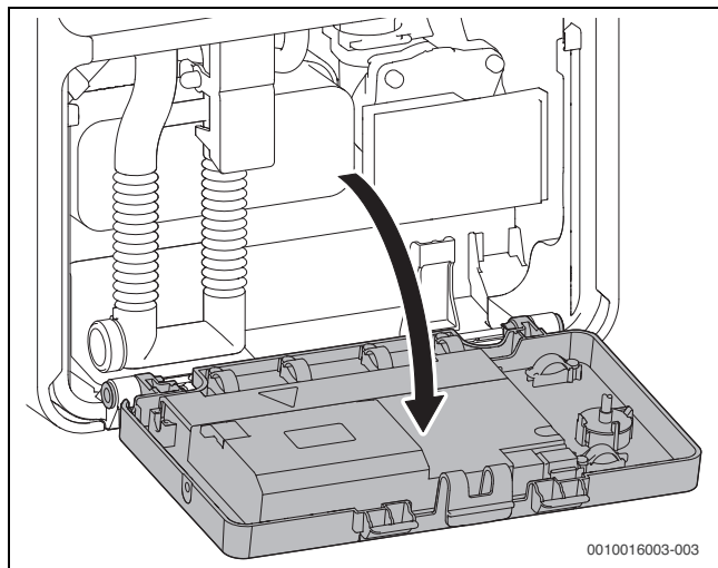
Fig. 26 Inclinar o sistema eletrónico para baixo
