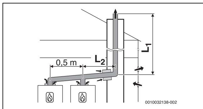
Fig. 18 Cascata com 2 aparelhos: Condução de gases queimados na condução de acordo com B 23p /B 53p com ar de admissão dependente do ar ambiente no aparelho
