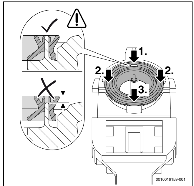
Fig. 54 Pressionar a vedação
