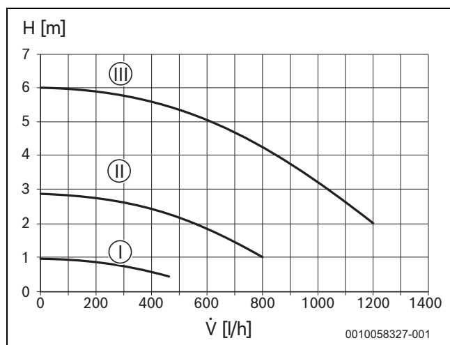
Fig. 33 Curva característica da bomba circuladora (pressão constante)
