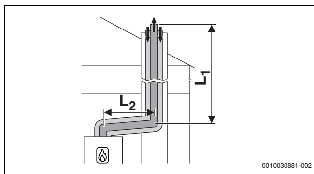
Fig. 8 Condução dos gases de escape para o exterior concêntrica de acordo com C_{33x} na condução
