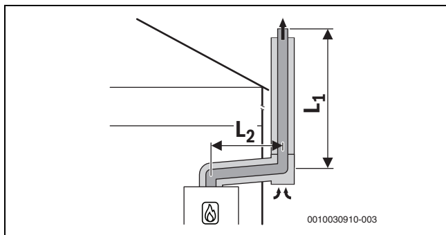
Fig. 13 Condução concêntrica dos gases queimados para o exterior de acordo com C 53x na parede exterior
