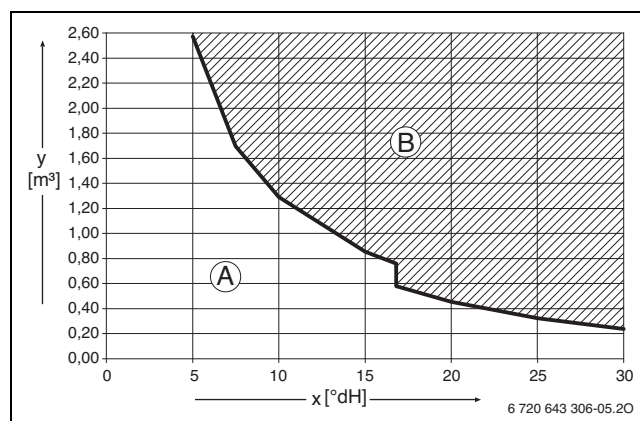
Fig. 19 Requisitos relativos à água de enchimento e à água adicional em °dH para instalações < 50 kW
