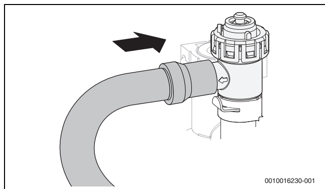
Fig. 23 Instalar a mangueira na válvula de segurança
