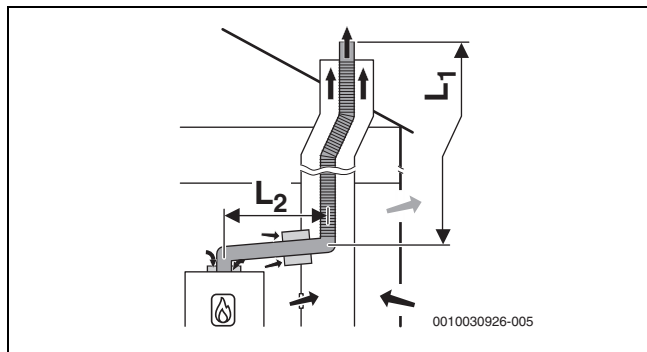
Fig. 15 Tubagem flexível de gases queimados no compartimento de acordo com B 53p com ar de admissão dependente do ar ambiente no aparelho e tubo de gases queimados simples no local de instalação; abertura de ventilação traseira no compartimento
