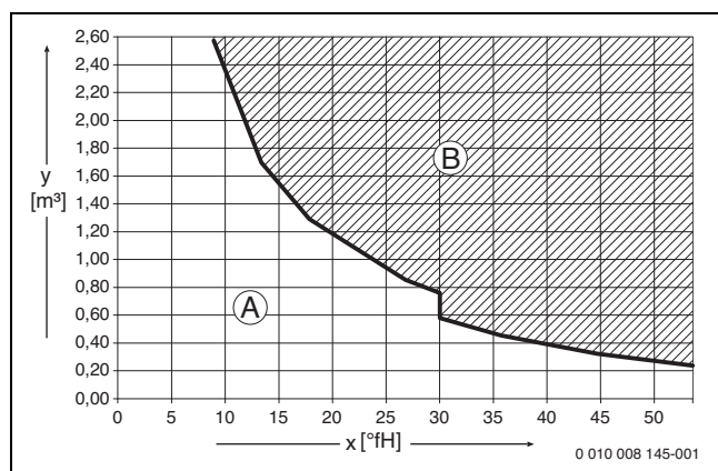
Fig. 20 Requisitos relativos à água de enchimento e à água adicional em °fH para instalações < 50 kW
