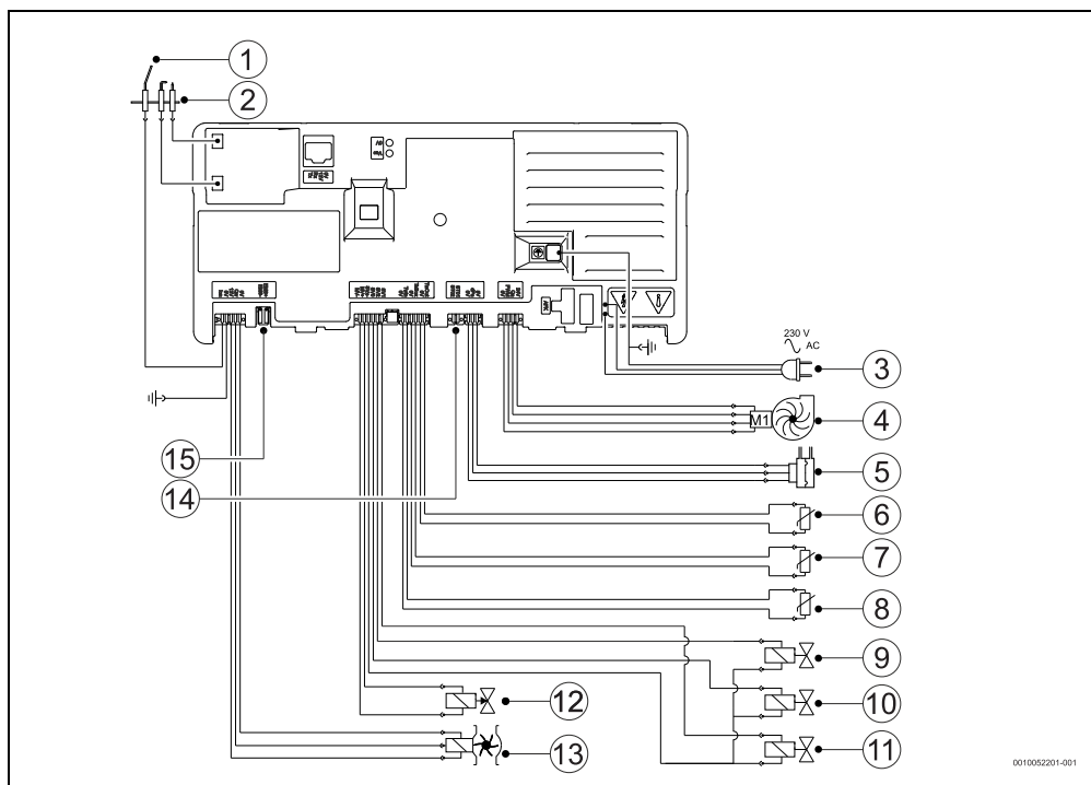
Fig. 32 Esquema elétrico
