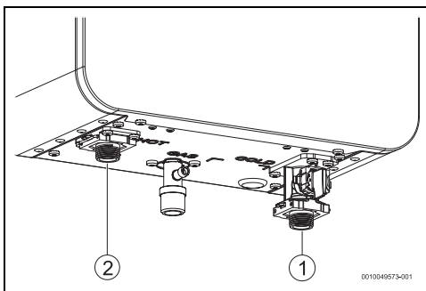
Fig. 22 Ligação da água
