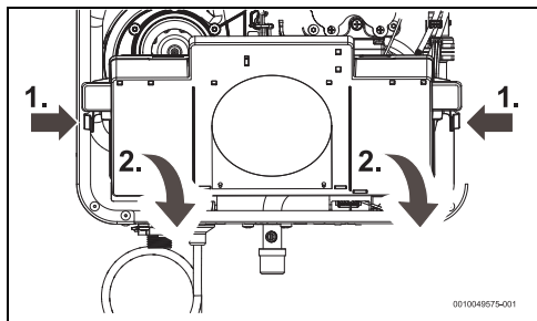
Fig. 27 Inclinar caixa de comando
