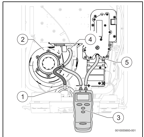
Fig. 29 Ligação ao ventilador, sensor de pressão e tomada de pressão de gás
