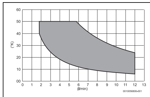
Fig. 33 Modelo 12 litros
