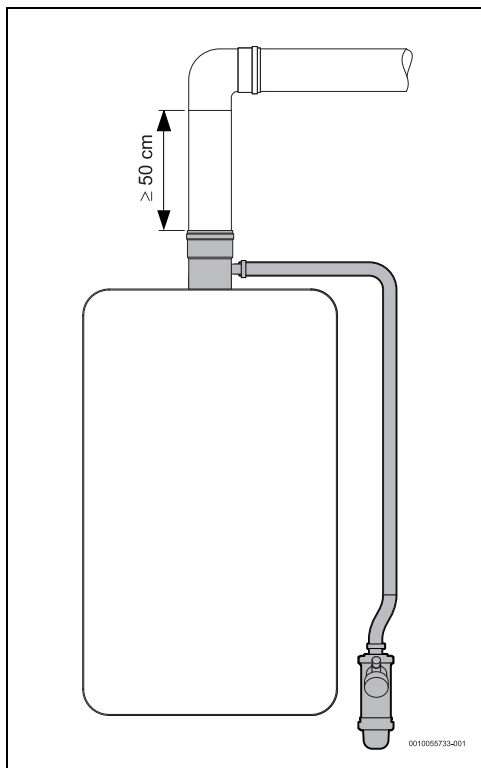
Fig. 17 Recolha de condensados (conduta horizontal)
