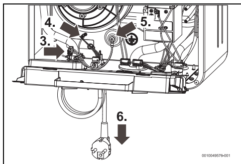
Fig. 28 Ligações cabo de alimentação
