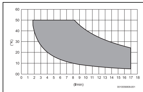
Fig. 35 Modelo 17 litros
