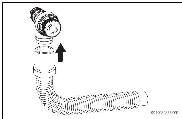
Fig. 19 Instalar a mangueira na válvula de segurança (aquecimento)
