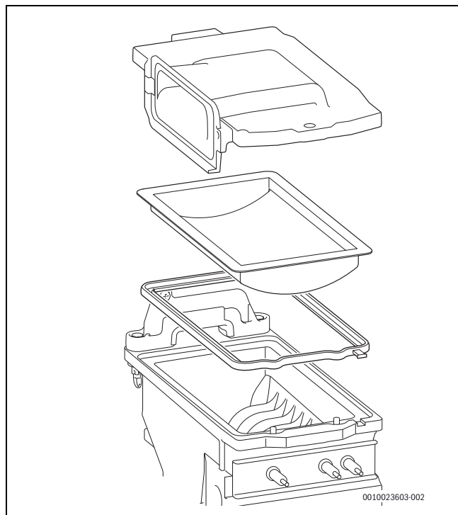
Fig. 40 Queimador
