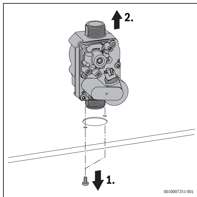
Fig. 54 Desmontar a válvula de gás
