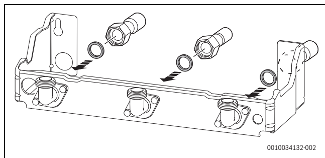
Fig. 18 Instalar os tubos com vedações na placa de ligação para montagem
