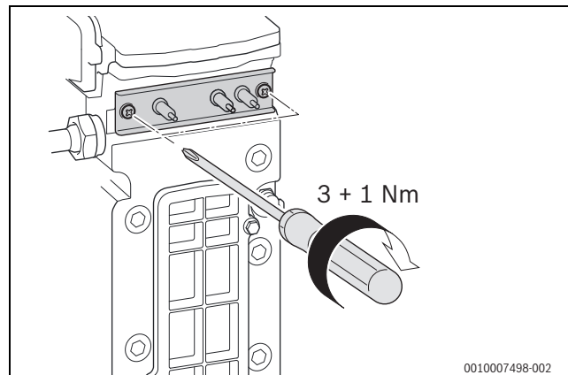
Fig. 37 Instalar o conjunto de elétrodos
