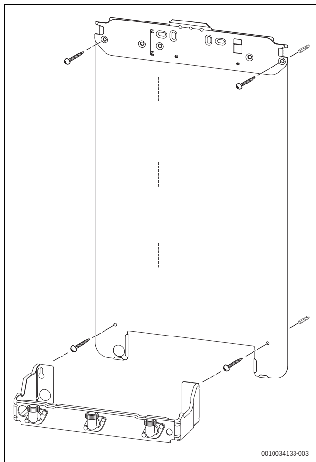
Fig. 17 Instalar a placa de fixação e a placa de ligação para montagem
