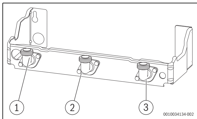
Fig. 25 Ligações do lado do gás e da água
