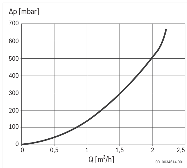
Fig. 55 Diagrama de perda de pressão
