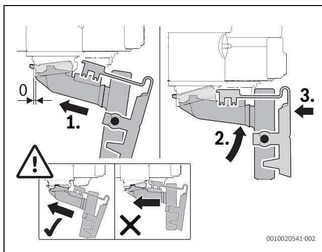
Fig. 51 Montar a recolha de condensados
