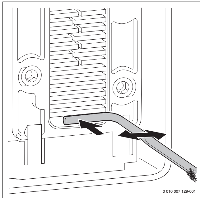
Fig. 47 Limpar a cuba de condensados
