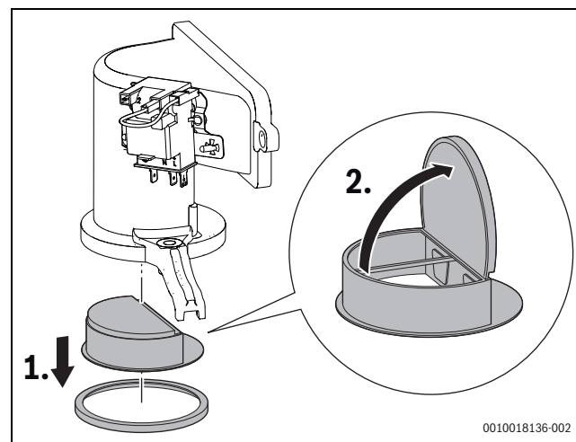
Fig. 43 Válvula antirretorno no dispositivo de mistura
