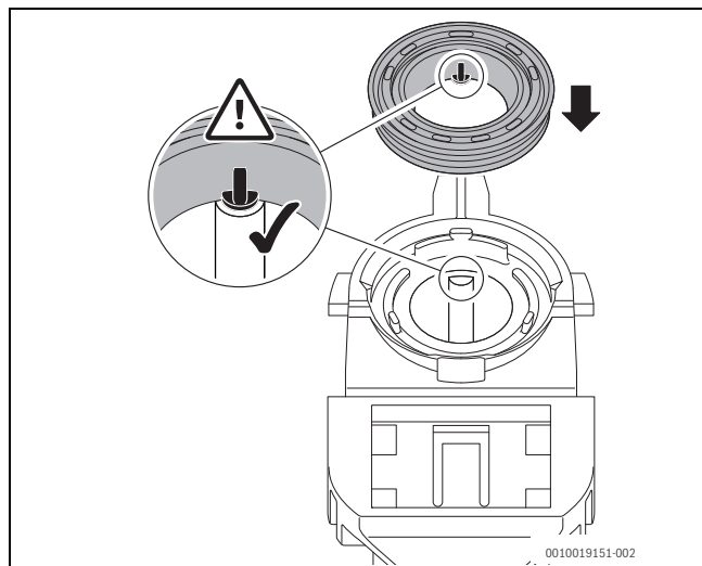
Fig. 49 Alinhar corretamente o novo vedante recolha de condensados
