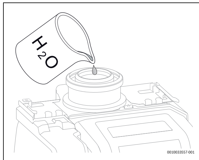
Fig. 23 Encher a recolha de condensados com água
