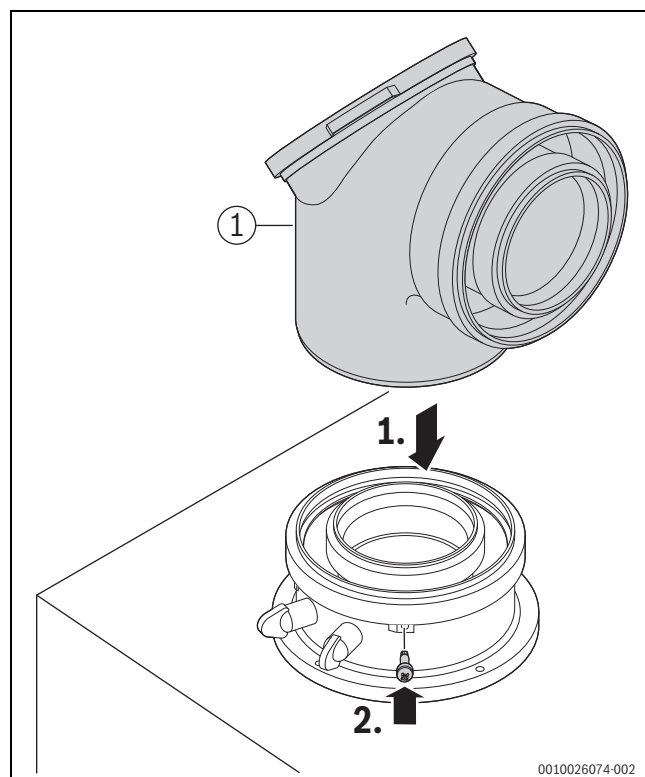
Fig. 24 Colocar e fixar os acessórios de exaustão com parafusos
