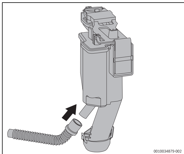
Fig. 20 Montar a mangueira de condensados na recolha de condensados
