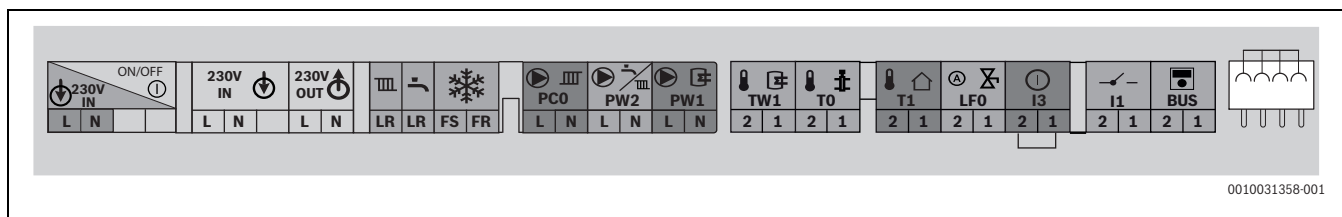
Fig. 28 Régua de bornes para os acessórios externos
