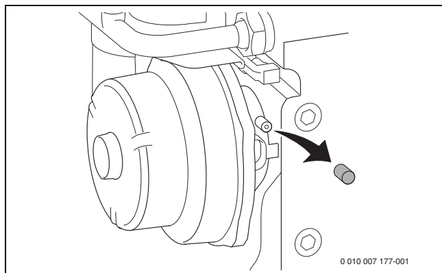
Fig. 44 Ponto de medição no dispositivo de mistura
