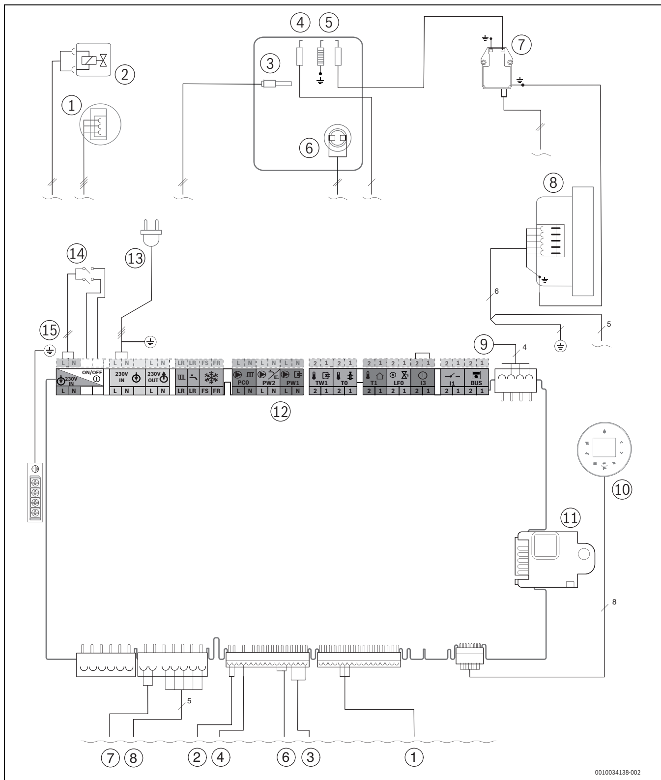
Fig. 56 Cablagem elétrica
