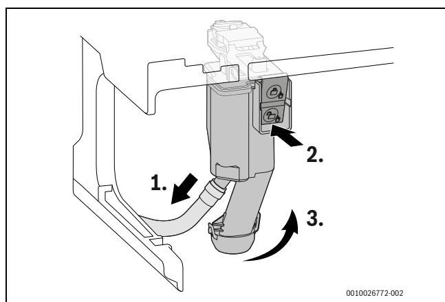
Fig. 48 Desmontar a recolha de condensados
