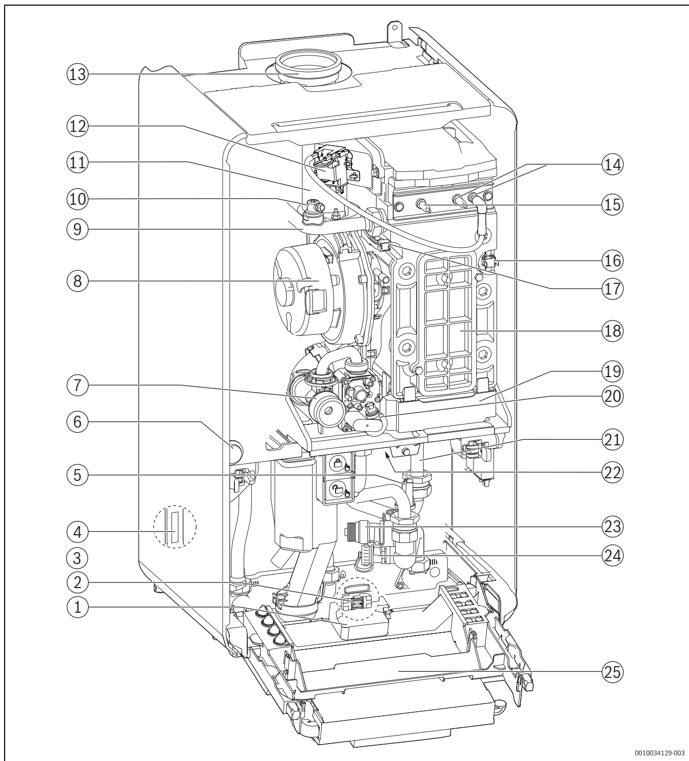
Fig. 4 Vista geral do produto
