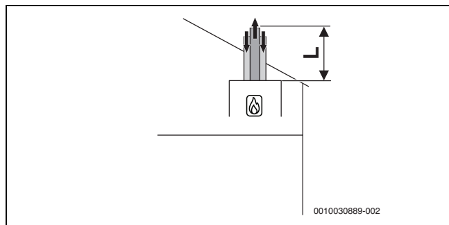
Fig. 8 Condução vertical e concêntrica dos gases de escape para o exterior de acordo com C 33x
