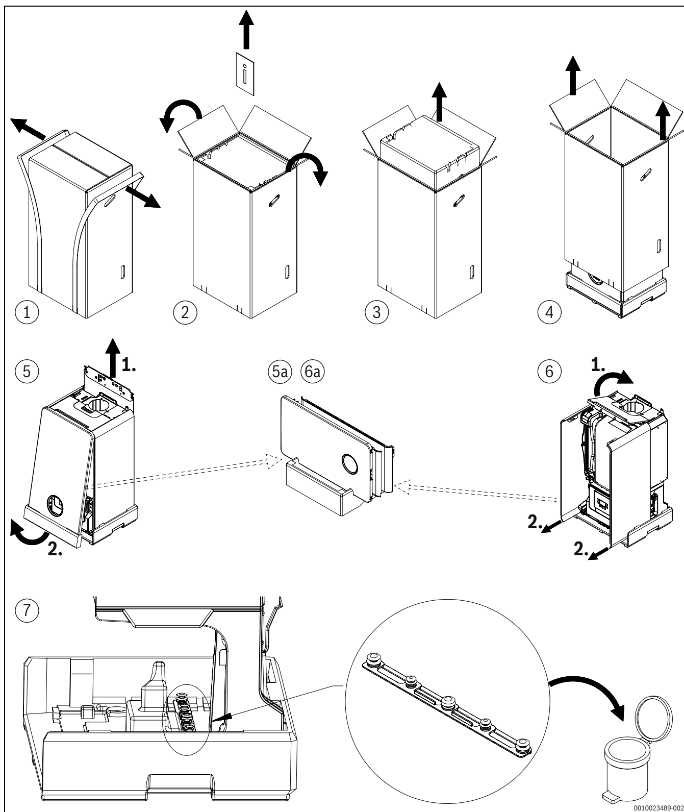
Fig. 16 Instrução para desembalar
