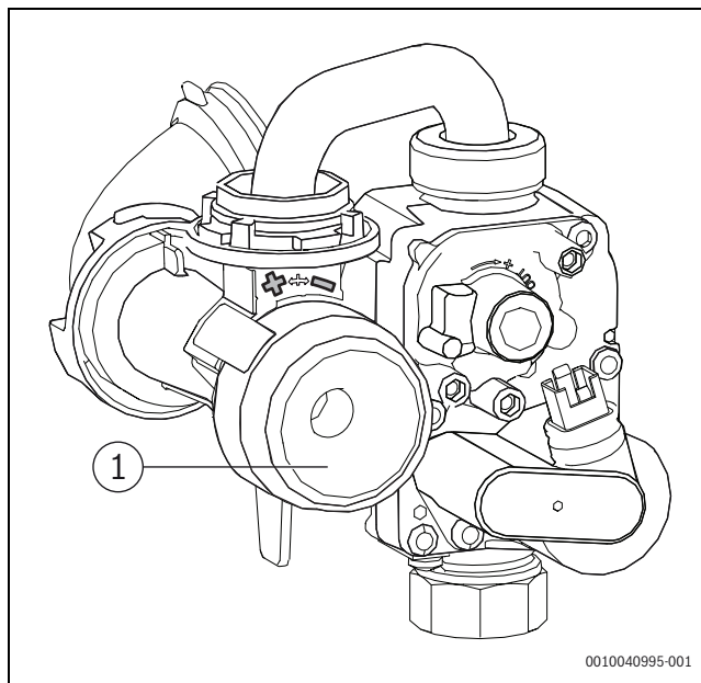
Fig. 32 Ajustar a relação gás/ar
