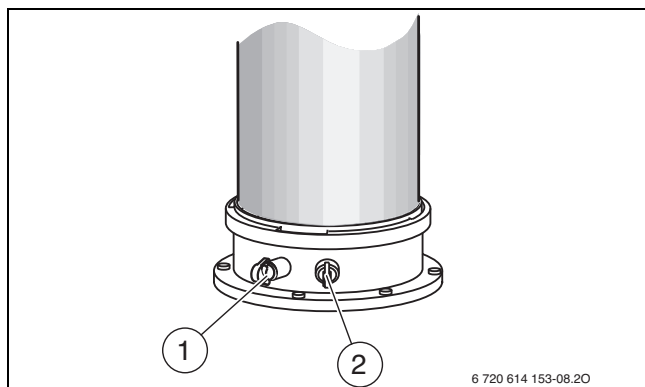
Fig. 36 Ponto de medição de gases queimados e ponto de medição do ar de combustão
