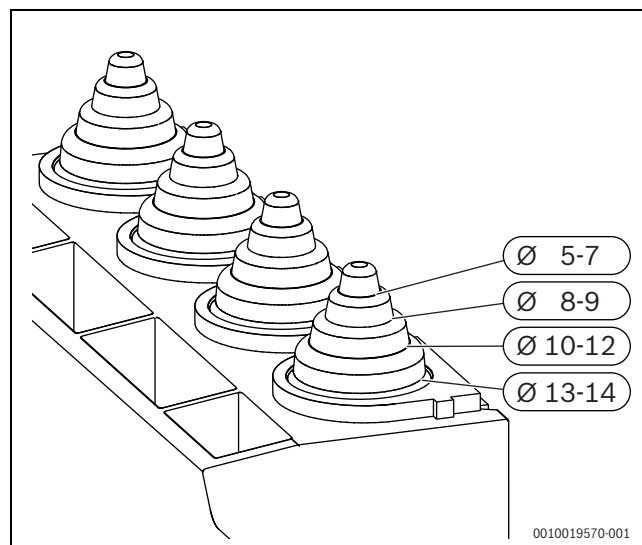
Fig. 27 Adaptar o dispositivo de redução de tração ao diâmetro do cabo
