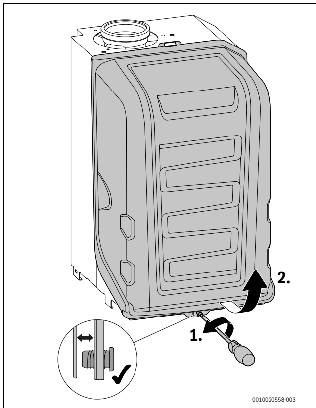
Fig. 31 Retirar a cobertura do queimador
