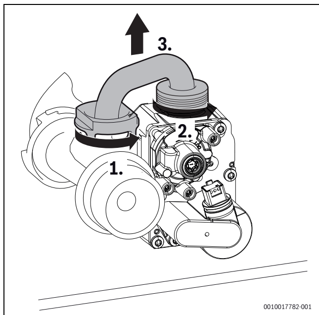
Fig. 52 Desmontar o tubo do gás
