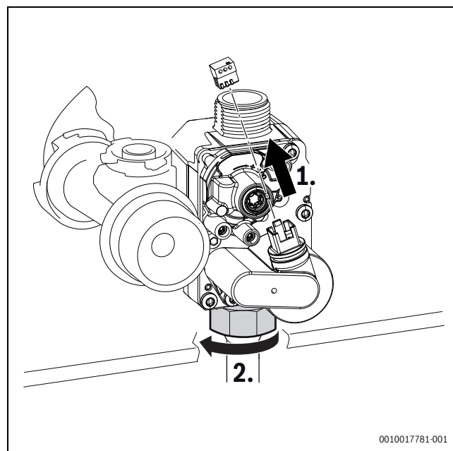
Fig. 53 Retirar a ficha e soltar a porca de aperto
