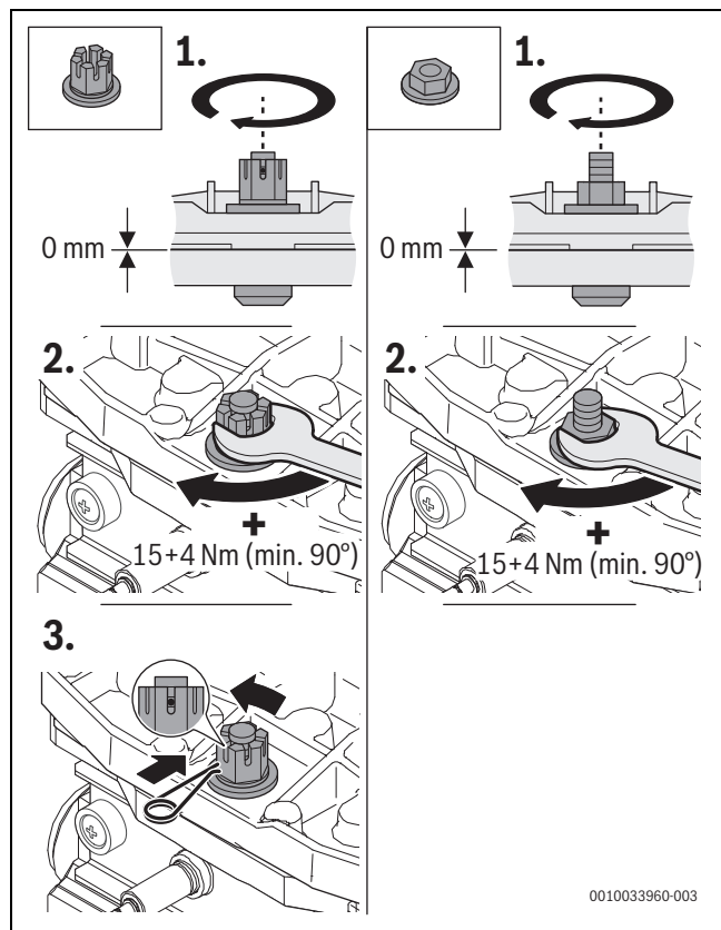
Fig. 41 Apertar a porca na tampa do queimador
