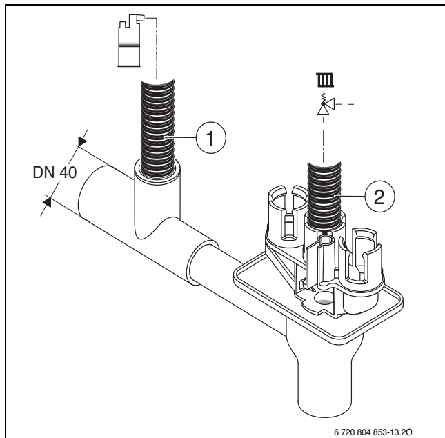
Fig. 21 Instalar a mangueira de condensados e a mangueira da válvula de segurança no sifão
