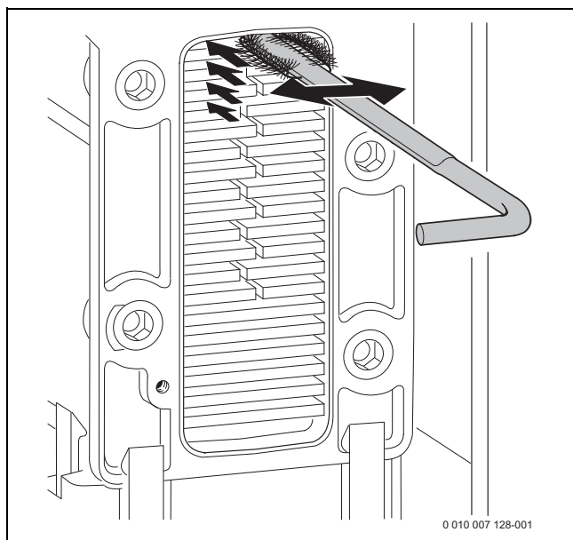
Fig. 45 Limpar o bloco térmico com a escova
