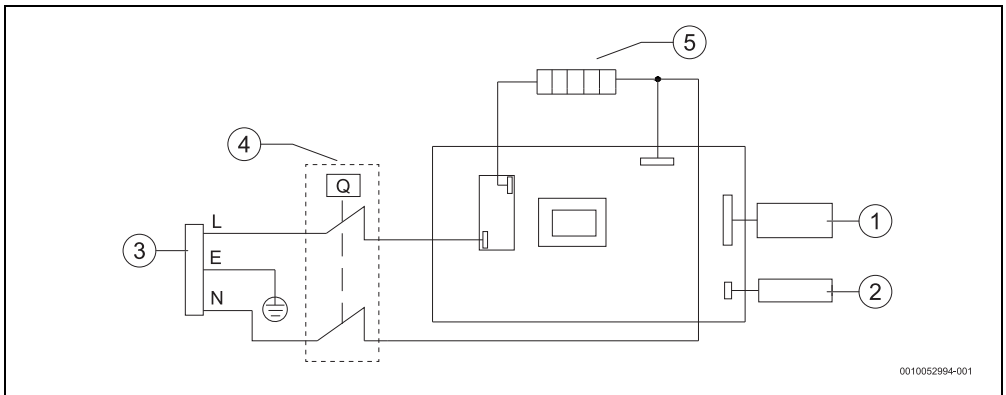
Fig. 12 Esquema de conexiones
