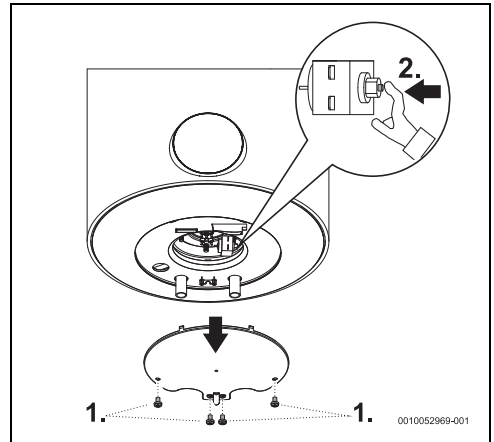
Fig. 11 Termostato de seguridad
