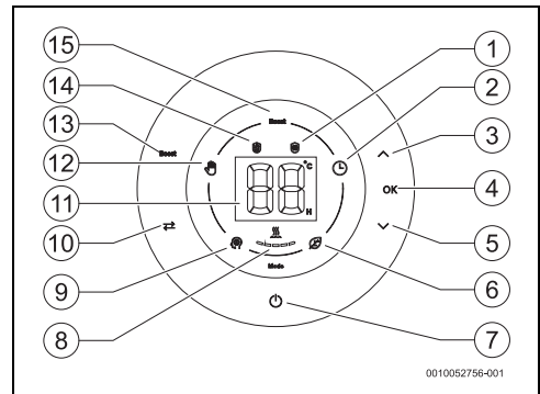
Fig. 4 Painel de comandos
