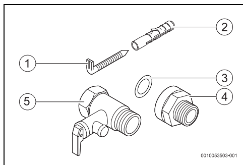
Fig. 1 Equipamento fornecido
