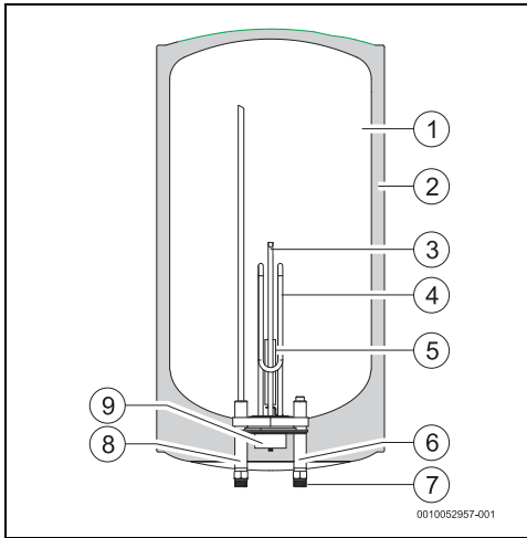
Fig. 3 Componentes del aparato
