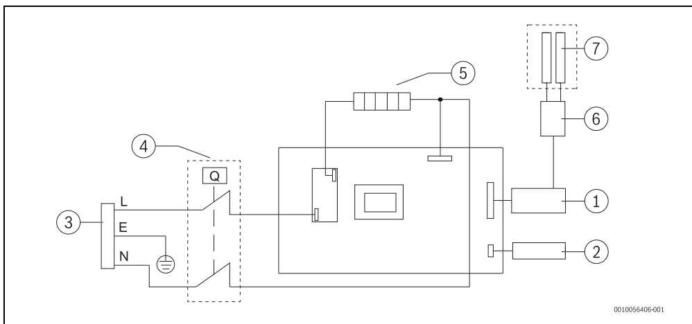
Fig. 12 Esquema de ligação
